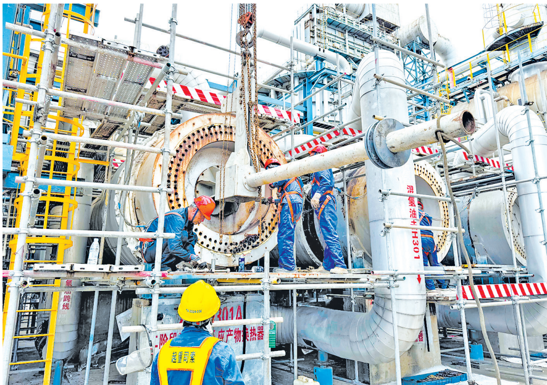
近日，福海创公司加氢裂化装置检修进入攻坚阶段，首台高压螺纹环锁紧换热器的螺纹环拆卸作业拉开序幕。（饶年清 摄）
