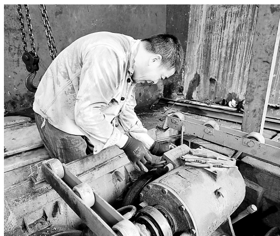
▲9月8日，为加快恢复西湖山、红一矿60多户住户居家用水，福建煤电红炭山物业站抢修队员们放弃午休，连续奋战6小时，确保职工家属在晚饭前可以正常用水。图为该站工作人员在水泵房更换水泵电机轴。（郑延玲 谢龙辉 摄）
