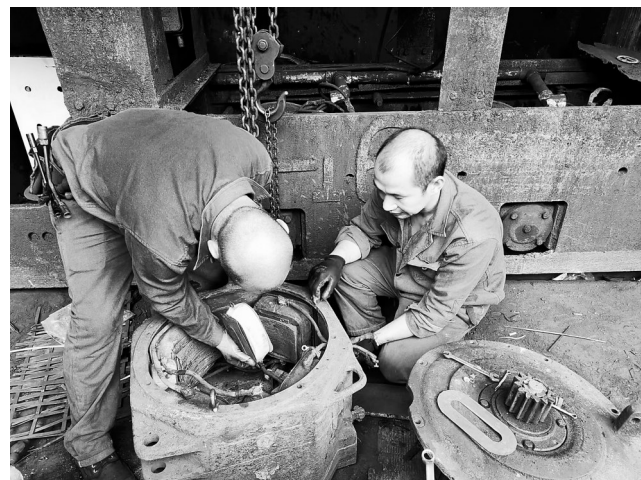
春节将至,为做好后勤保障工作,福建煤电公司翠屏山煤矿机电队组织人员对部分简易电气设备进行自检自修,及时维修或更换相关配件,保证正常的生产使用需求。图为该矿机电队人员在更换损坏的磁极线圈。(邱素梅 摄)
